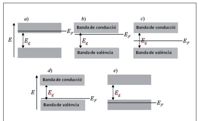
FIGURA 3. Diagrama d'energia de: a) un metall amb una funció de treball petita; b) un semiconductor de tipus n ; c) un aïllant; d) un semiconductor de tipus p ; e) un metall amb una funció de treball gran.
